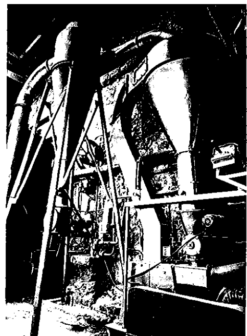
De maalinrichting 1961.
